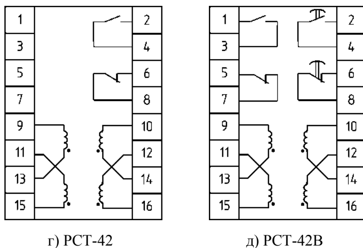
Рисунок Г.1 –Схемы подключения реле (для исполнений по выходным контактам 1з1р)
